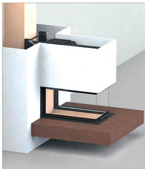
Cadre de support fixé à la plaque de fond pour une installation comme « foyer suspendu »
