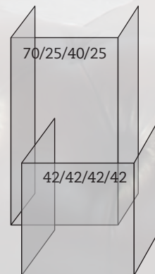
Spécification de format de porte hauteur x largeur côté x largeur front x largeur côté en cm
