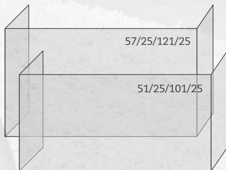
Spécification de format de porte hauteur x largeur côté x largeur front x largeur côté en cm
